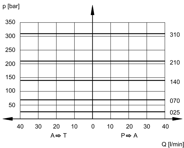
EINGESTELLTER DRUCK p_{max} = f(Q)
