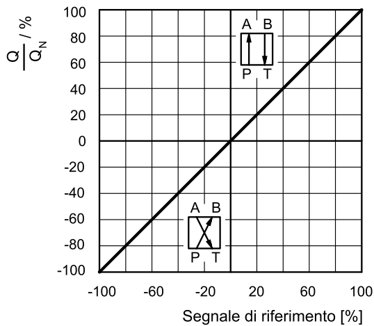
CARATTERISTICA PORTATA/RIFERIMENTO
