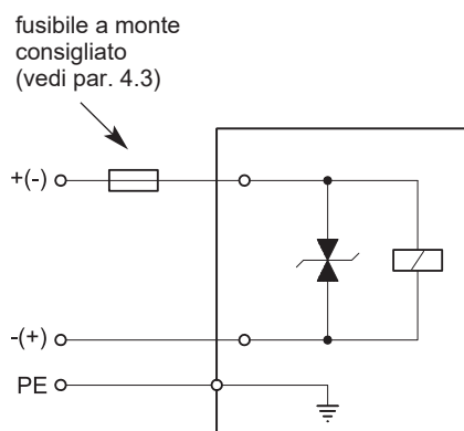
Bobina CC
