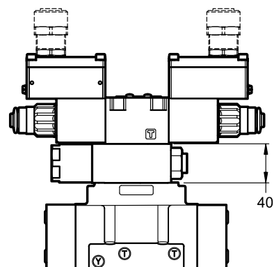
DSP*K*-/Z*
