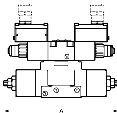
DSP*K*-/C
