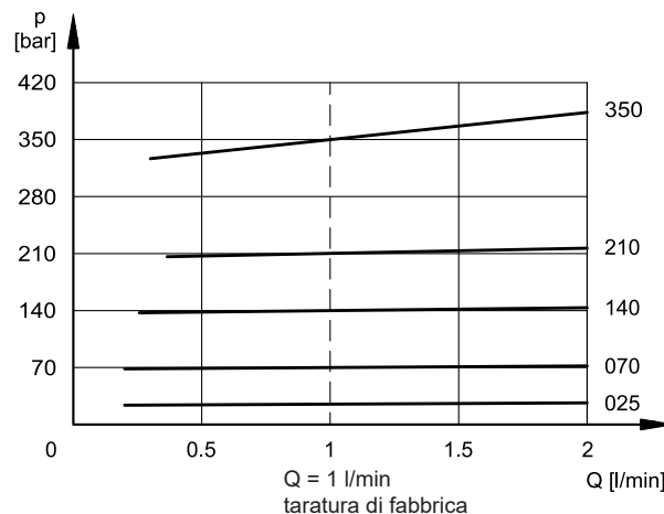
VARIAZIONE PRESSIONE p_{max} = f(Q)
