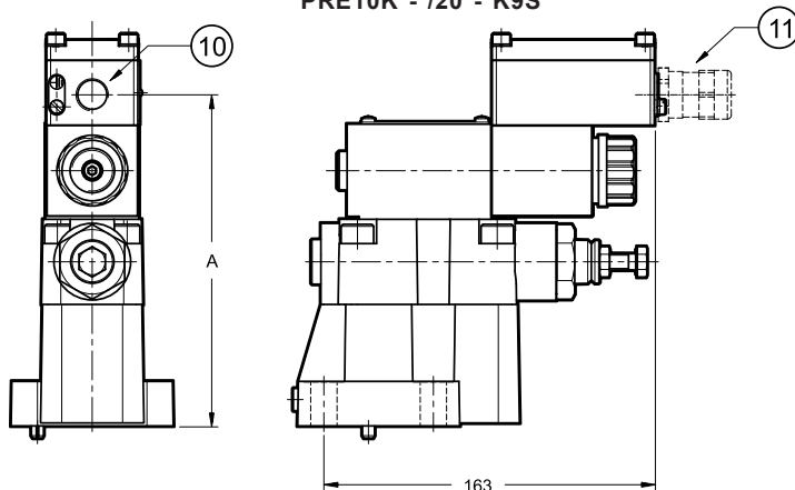
PRE10K*-/20*-*K9S*
