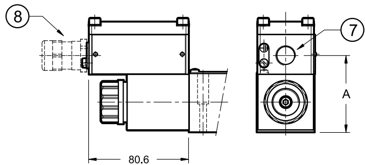
PDE3K*-/10*-*K9S*
