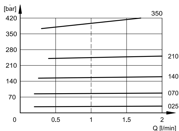
VARIAZIONE PRESSIONE p_{\text{max}} = f(Q)
