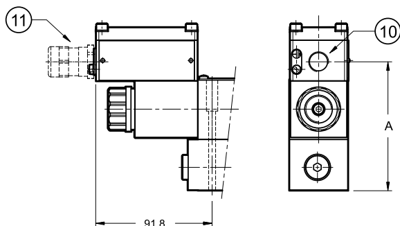
PRE3K*-/20*-*K9S*
